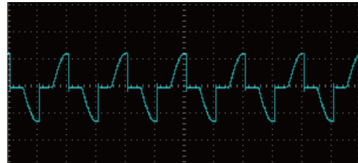
后沿相位调光
