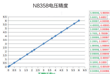
▲ 电压精度对比
