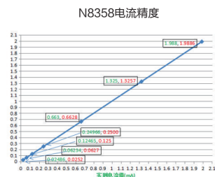
▲ 电流精度对比
